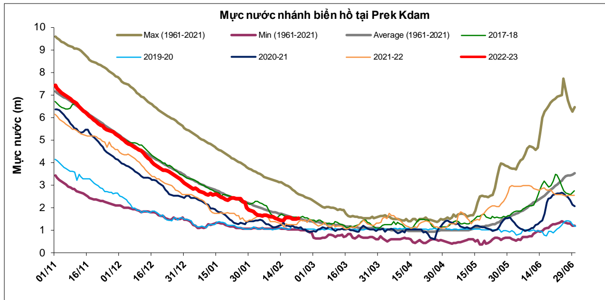
Hình 1. Diễn biến mực nước trạm Prek Kdam - Biển hồ, cập nhật ngày 22/2/2023
