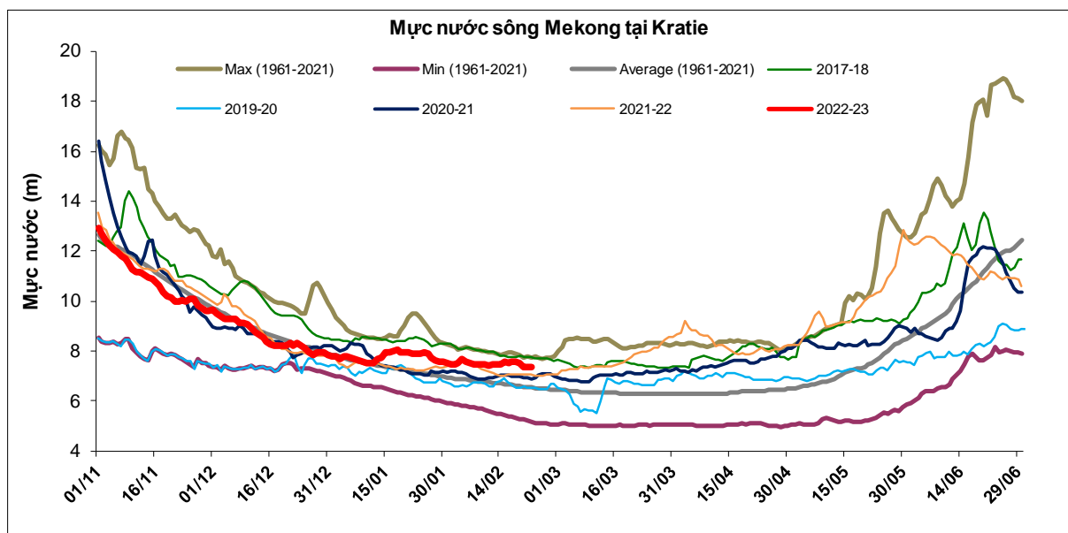
Hình 3. Diễn biến mực nước về qua trạm Kratie, cập nhật ngày 22/2/2023
