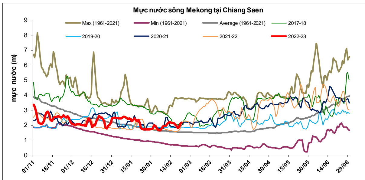
Hình 2. Diễn biến mực nước tại Chiang Saen –Thái Lan, cập nhật 22/2/2023
